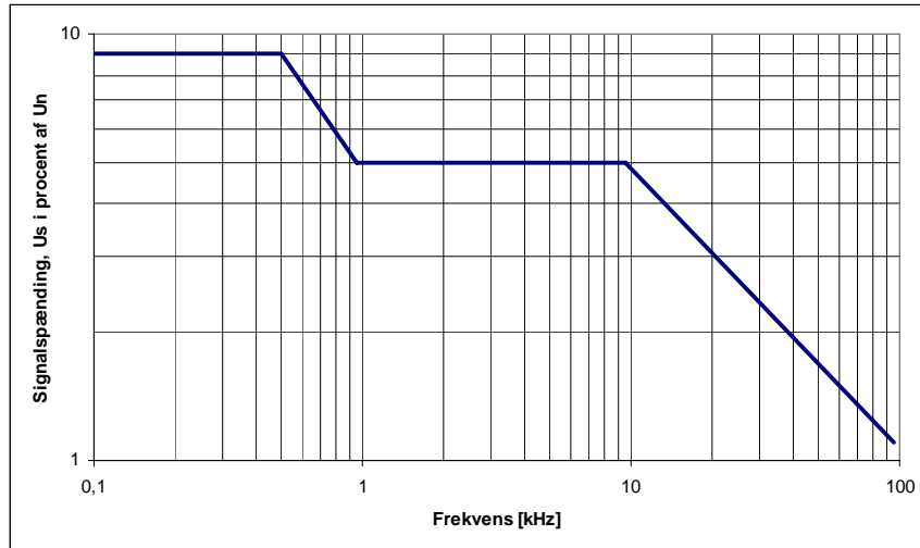
Figur 1: Maksimale signaltransmissionsspændinger
